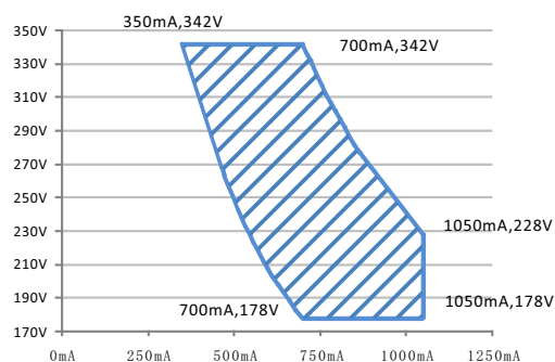
◎ XLG-240-L-DA2
