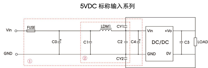
图 5 注：图 5 中第①部分用于 EMC 测试；第②部分用于 EMI 滤波，可依据需求选择。
