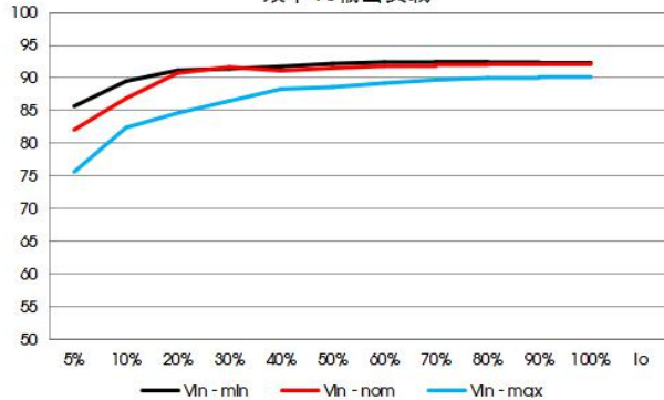
VCF4824EBO-120W(F)R3-N 效率VS输出负载
