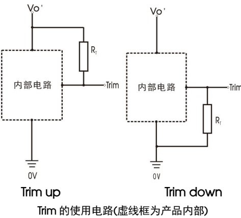
Trim 的使用电路(虚线框为产品内部)
