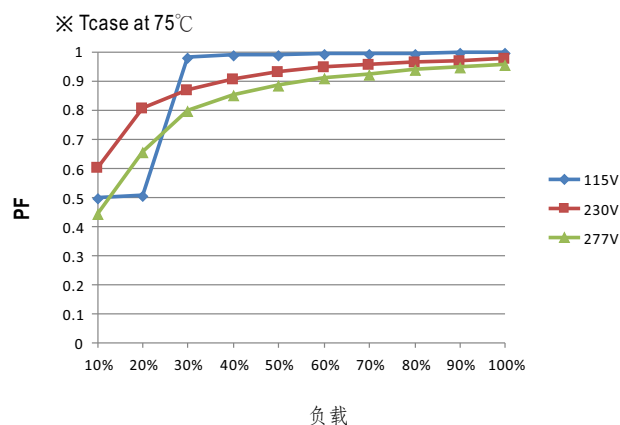
■ 功率因素特性曲线
