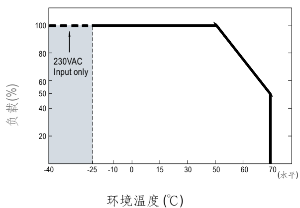
■ 减额曲线
