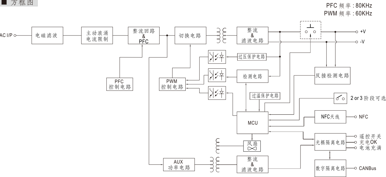
■ 方框图
