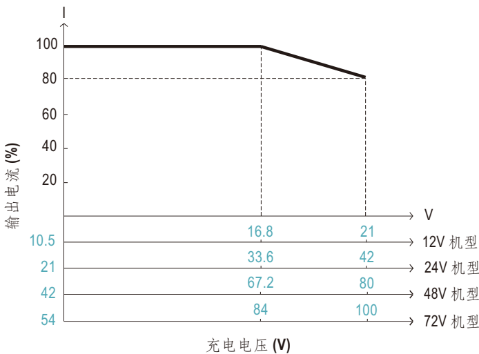
■ 减额曲线
