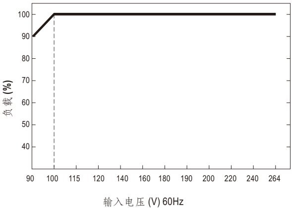
■ 静态特征曲线
