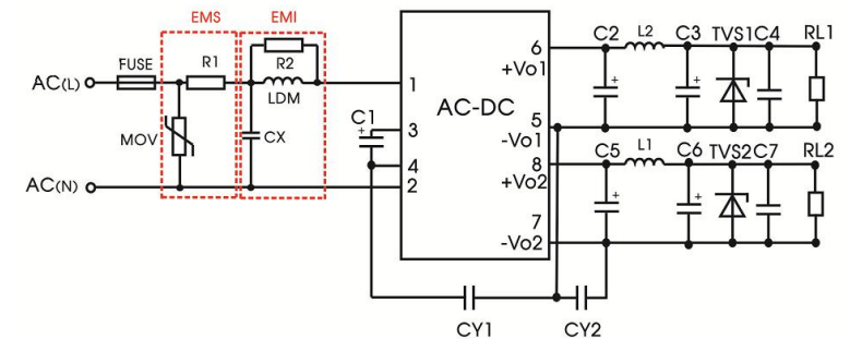
推荐电路 3
