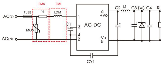
推荐电路 4
