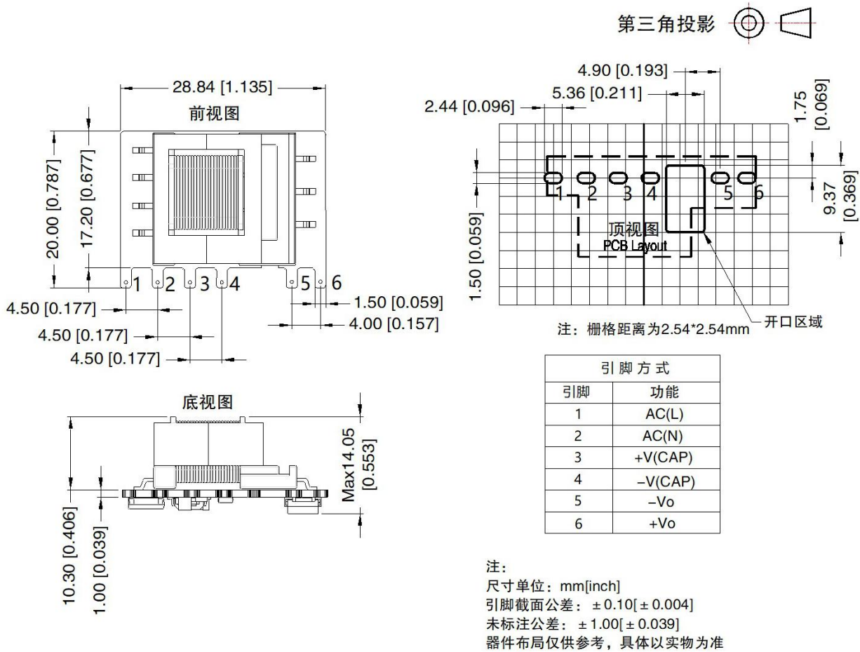
LS10-13BxxR3P 系列外观尺寸图
