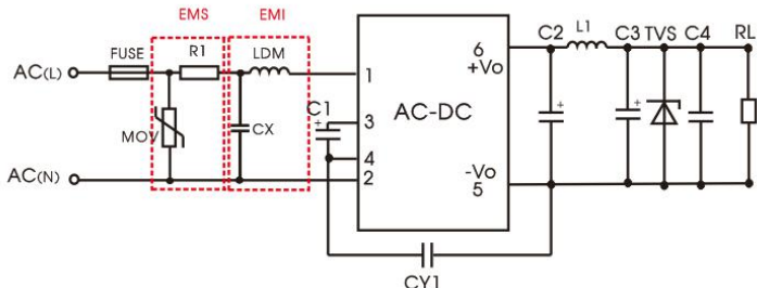
推荐电路 3
