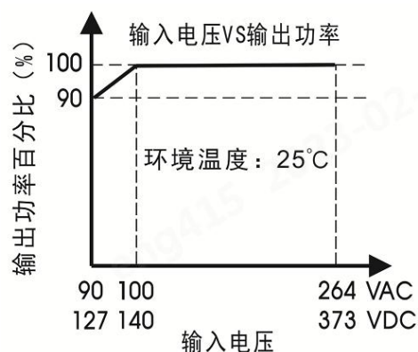
LOF350-20Bxx-CZ 输入电压降额
