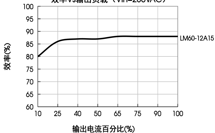
效率Vs输出负载 (Vin=230VAC)
