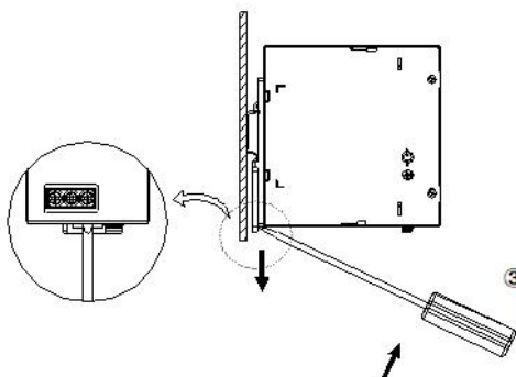
接/拆线步骤⑤-⑥
